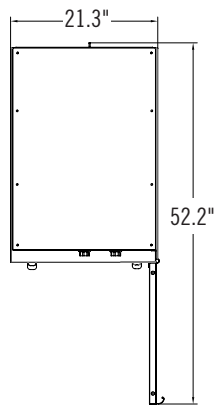
TOP VIEW / DOOR OPEN 90°
